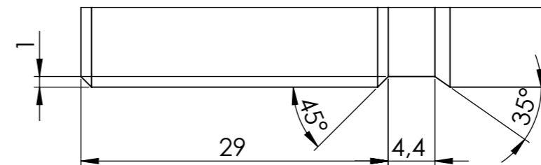
DETAIL A 2:1
