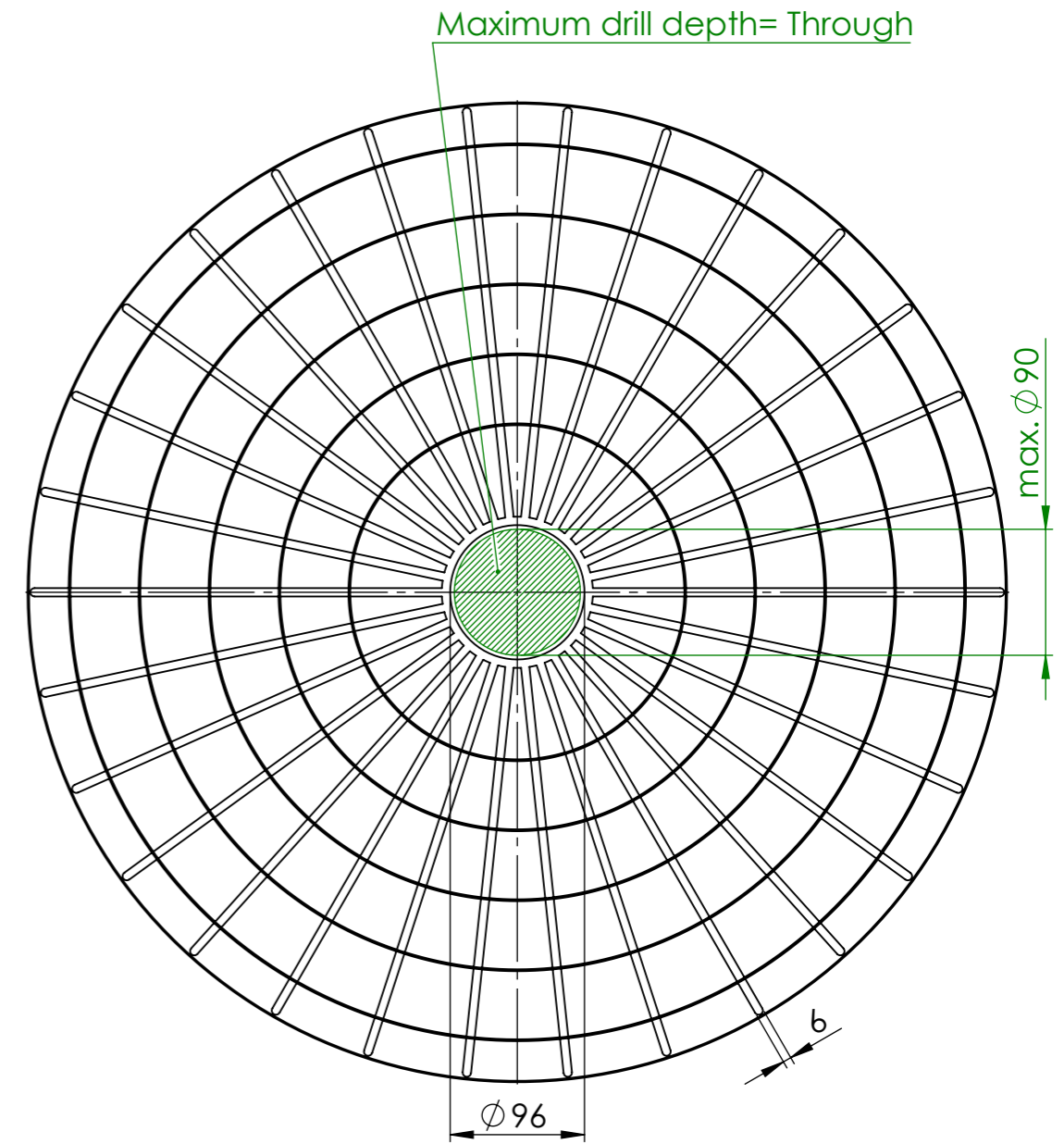
DETAIL A 2:1
